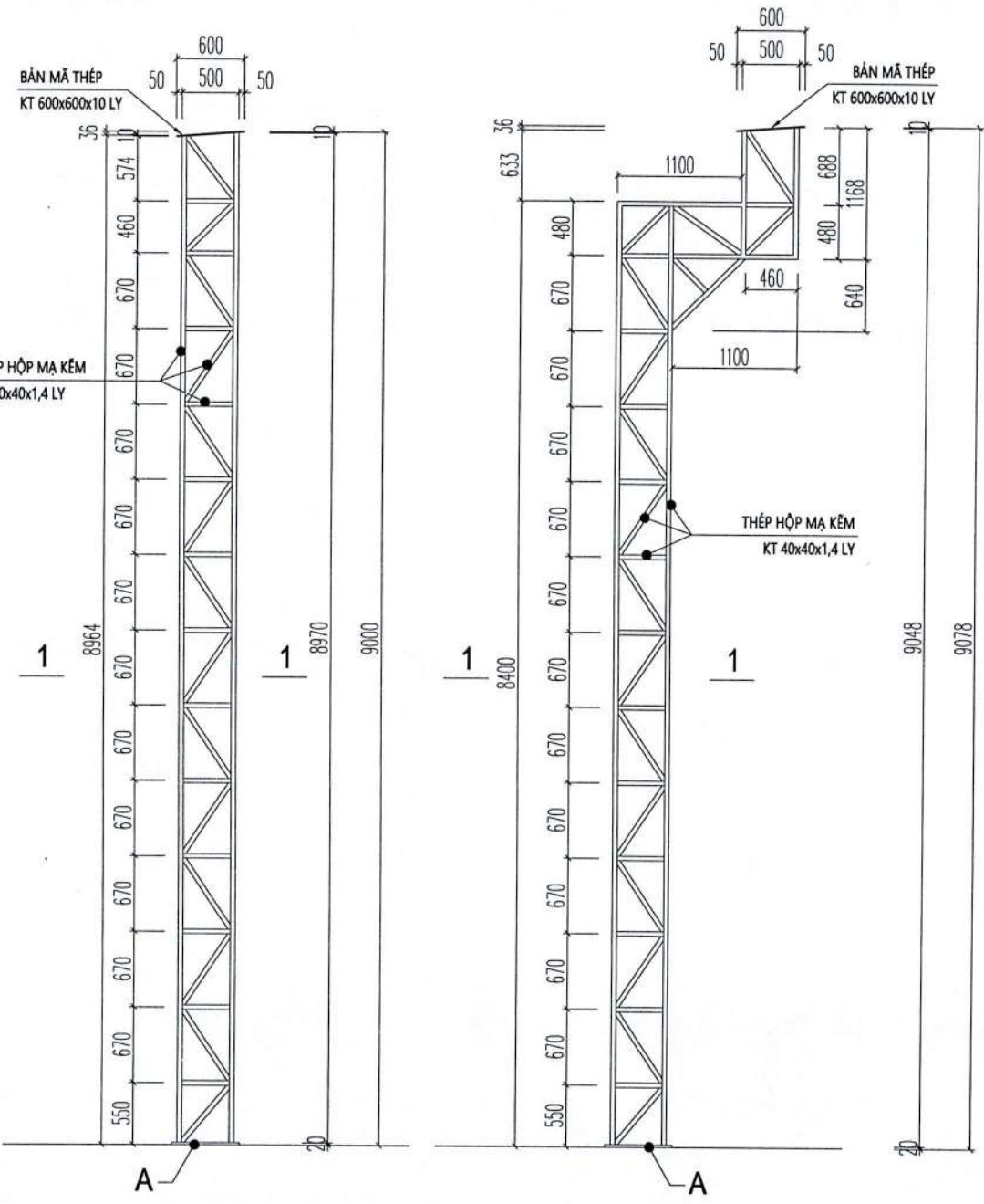
CHI TIẾT CỘT C6 (SỐ LƯỢNG: 02)
