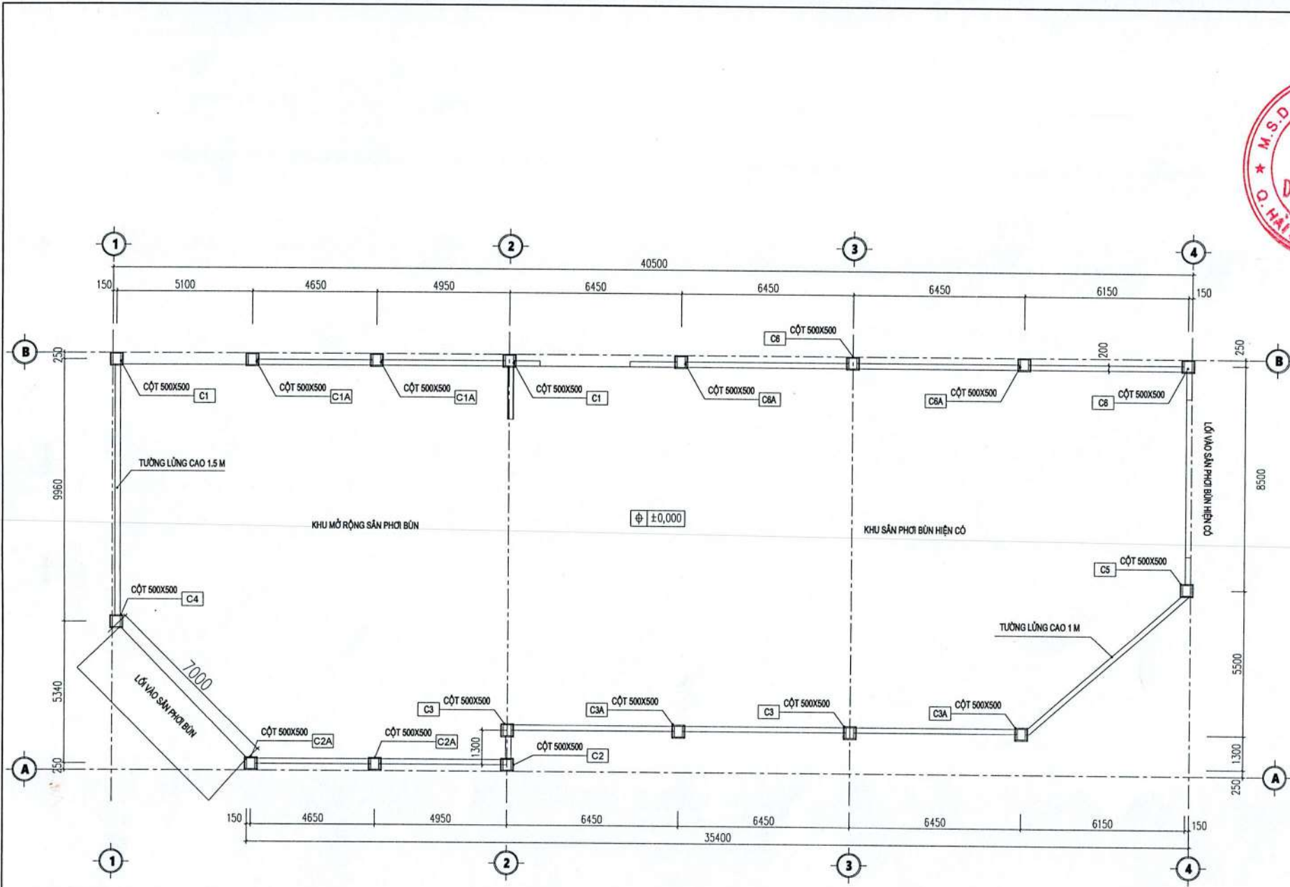
MẶT BẰNG CỘT MÁI CHE
