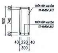
MẶT CẮT DẠM D3 (SỐ LƯỢNG: 01)
