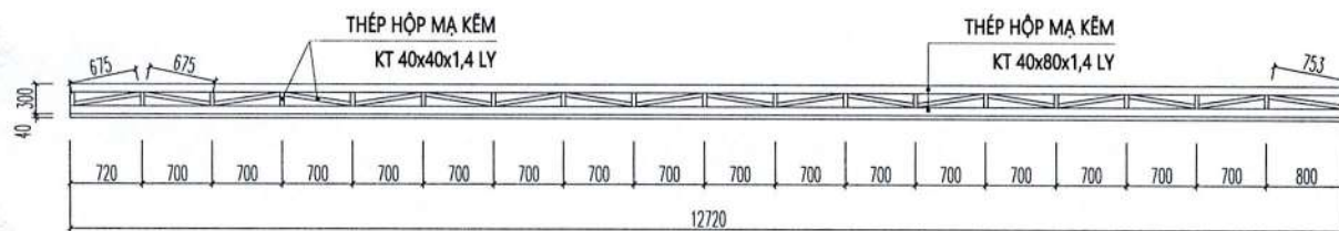
CHI TIẾT KÈO K2
