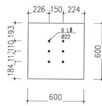
CHI TIẾT A
