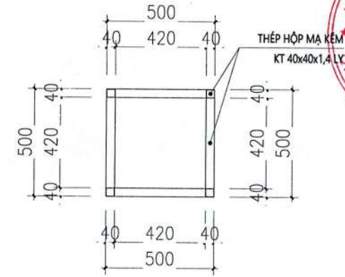
MẶT CẮT 1-1
