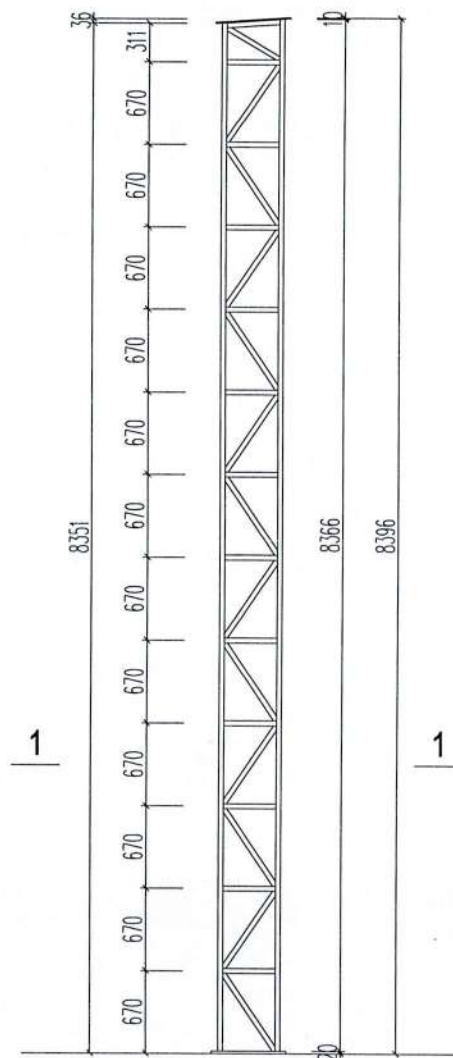
CHI TIẾT CỘT C5
