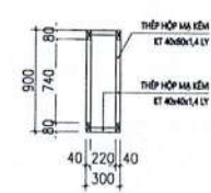
MẶT CẮT DẠM D5 (SỐ LƯỢNG: 04)
