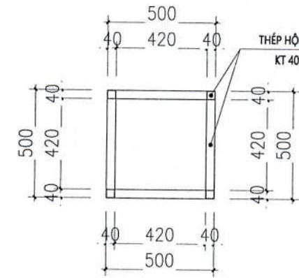
MẶT CẮT 1-1
