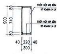
MẶT CẮT DẠM D1 (SỐ LƯỢNG: 01)
