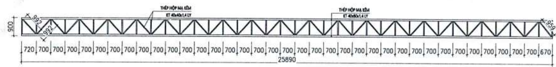
MẶT ĐỨNG DẠM D4 (SỐ LƯỢNG: 01)
