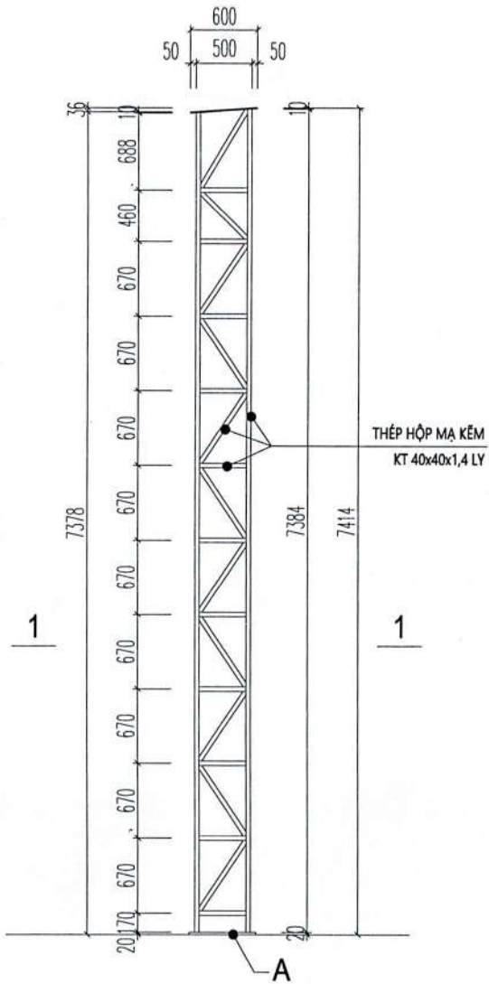
CHI TIẾT CỘT C2
