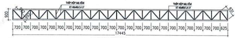
MẶT ĐỨNG DẠM D2 (SỐ LƯỢNG: 03)
