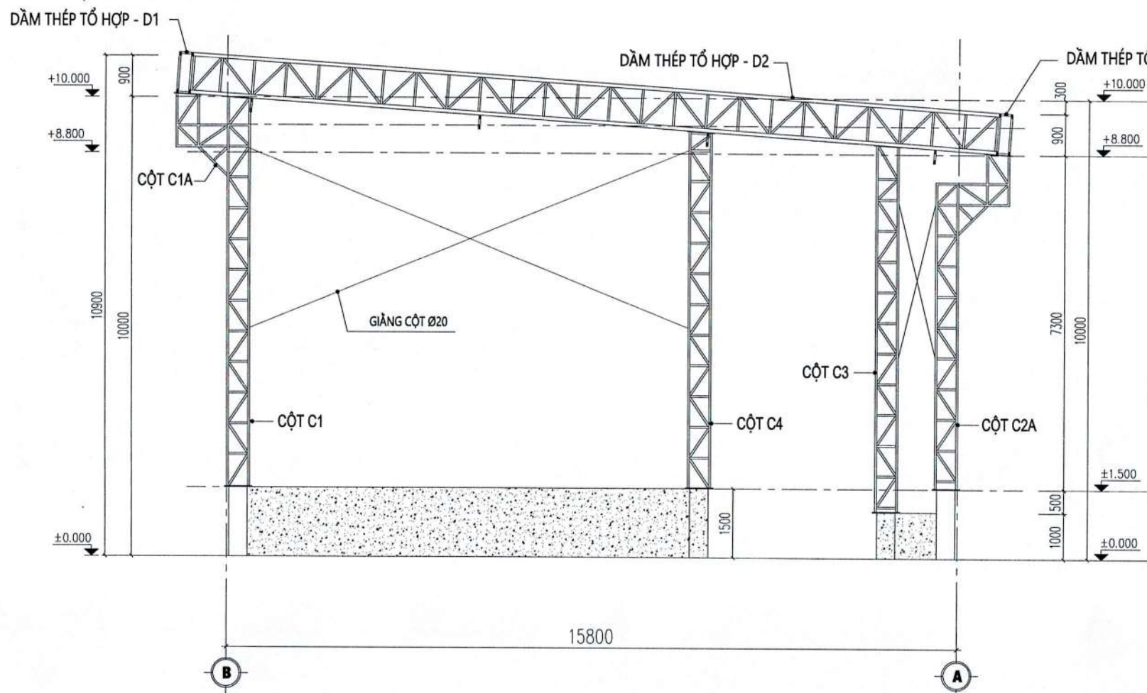
MẶT ĐỨNG TRỤC B-A
