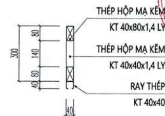
MẶT CẮT KÈO K1
