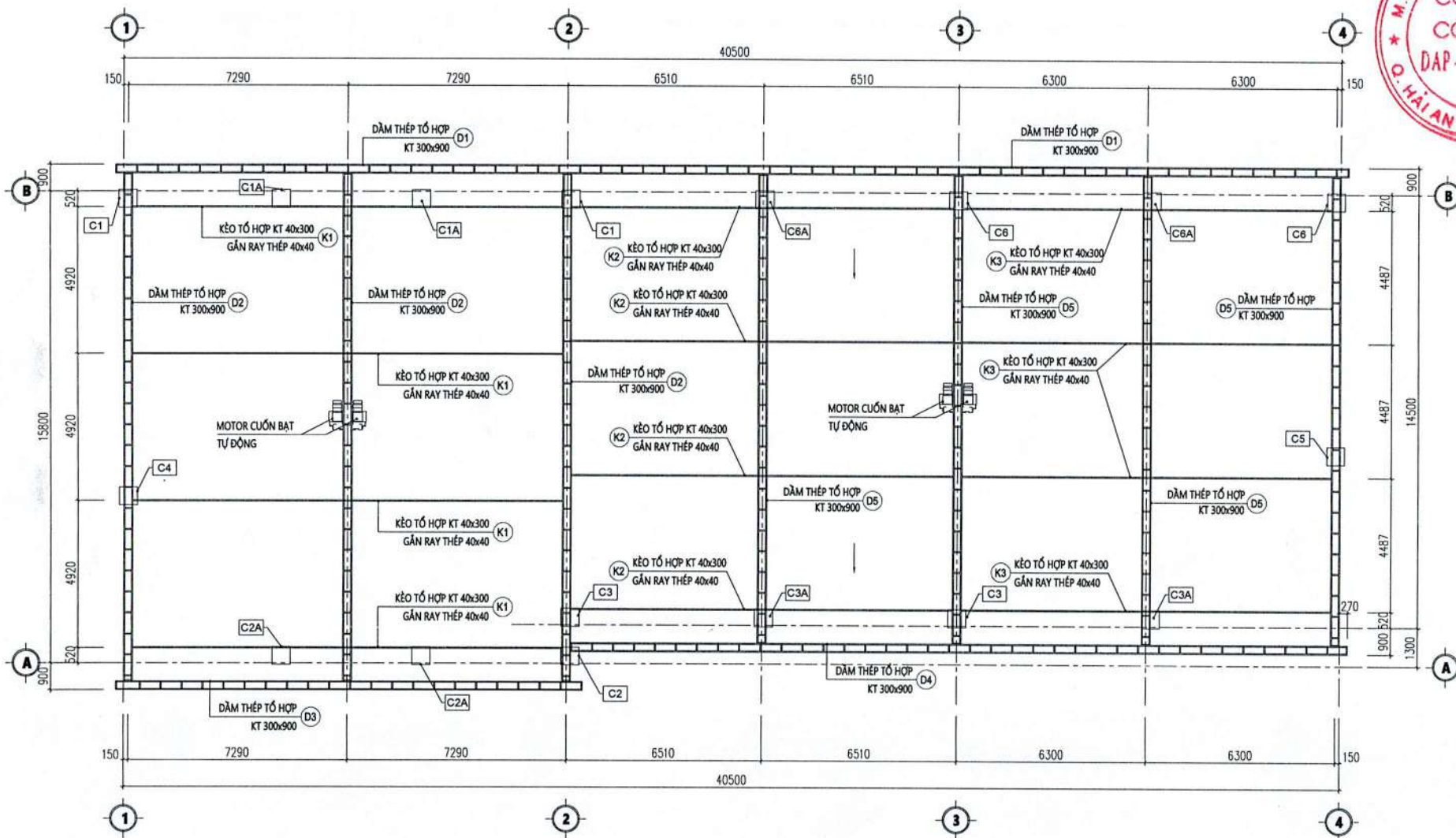
MẶT BẰNG MÁI CHE
