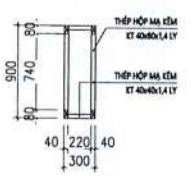
MẶT CẮT DẠM D4 (SỐ LƯỢNG: 01)
