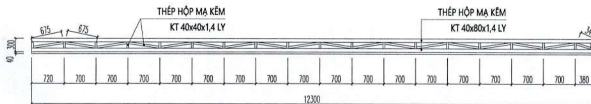
CHI TIẾT KÈO K3
