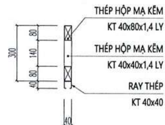
MẶT CẮT KÈO K2
