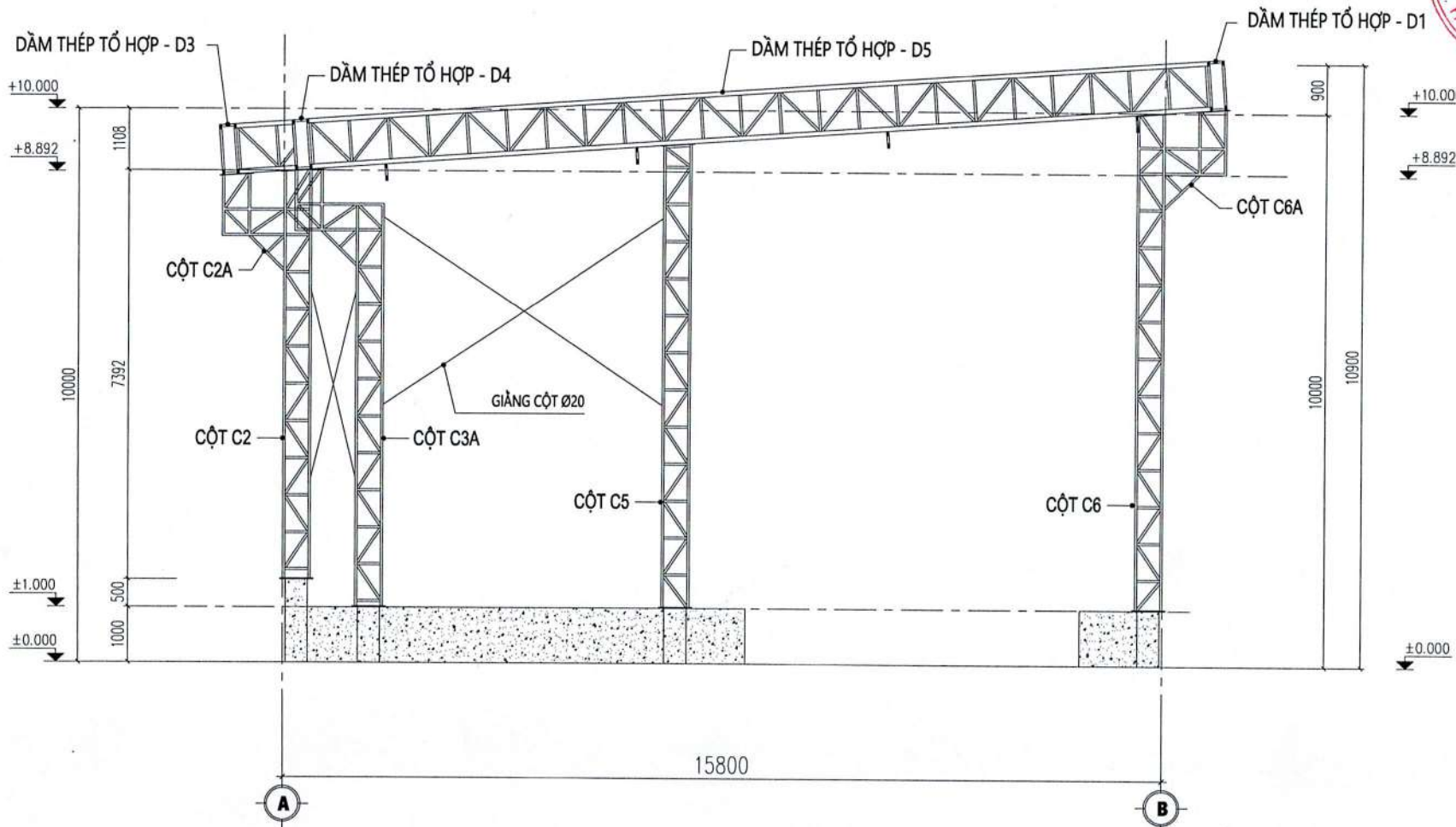
MẶT ĐỪNG TRỤC A-B
