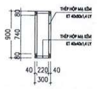
MẶT CẮT DẠM D2 (SỐ LƯỢNG: 03)
