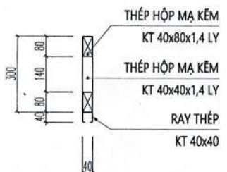
MẶT CẮT KÈO K3
