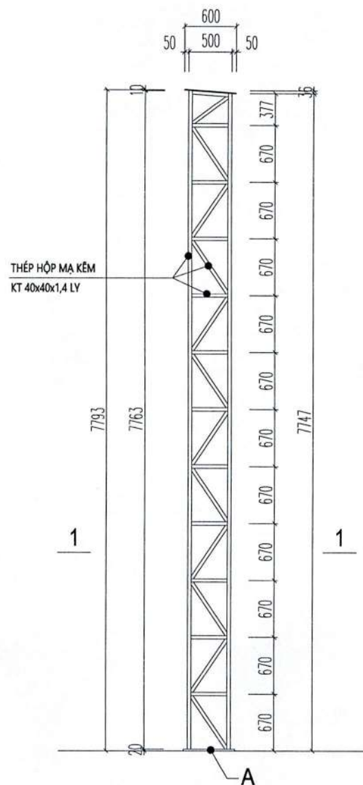
CHI TIẾT CỘT C4
